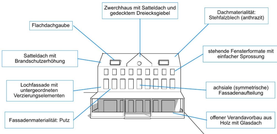
Abbildung 5: Skizze Bautyp 1
