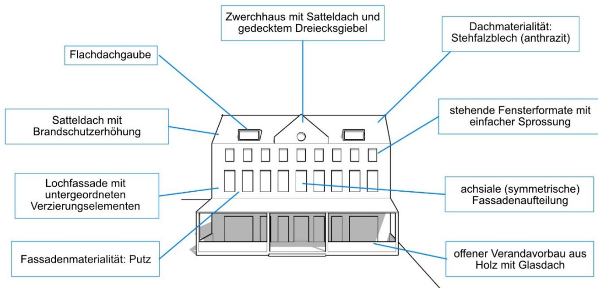
Abbildung 5: Skizze Bautyp 1
