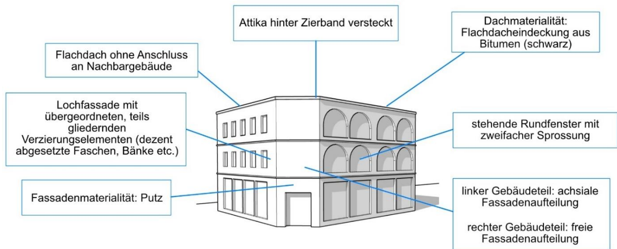
Abbildung 8: Skizze Bautyp 4
